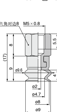
ZP2-TB08MB□□-B5
