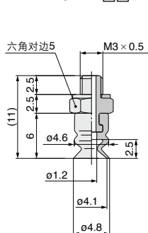
ZP2-TB04MB□□-A3
