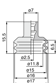
ZP2-B30J□
