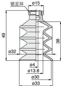
ZP2-B30J□
