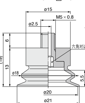
ZP2-TB20MB□□-H5
