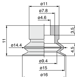
ZP2-B15MB□
