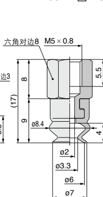
ZP2-TB06MB□□-B5
