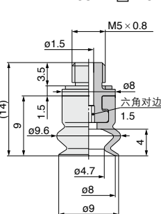
ZP2-TB08MB□□-H5
