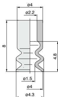
ZP2-04ZJ□
