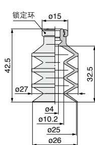
ZP2-B25J□
