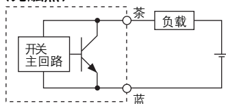
2线式 (无触点)
