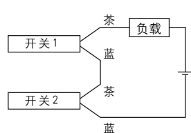
2线式的场合·2个AND连接
