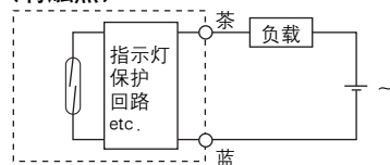
2线式 (有触点)
