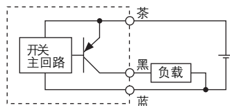
无触点3线式, PNP
