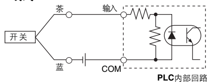
2线式
