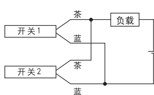
2线式的场合·2个OR连接
